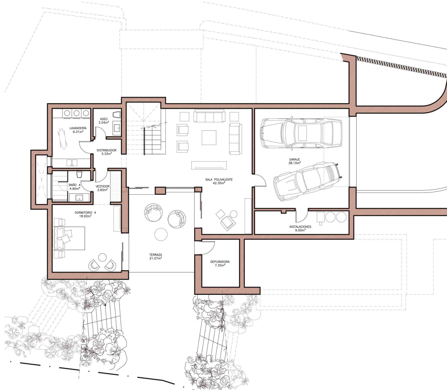
PLANTA SOTANO
